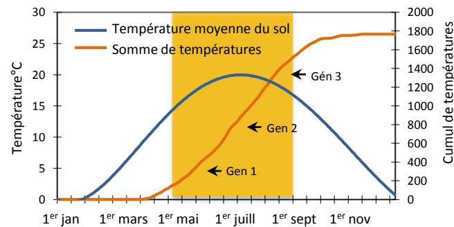
Développement des générations de nématodes en fonction de la température du sol
